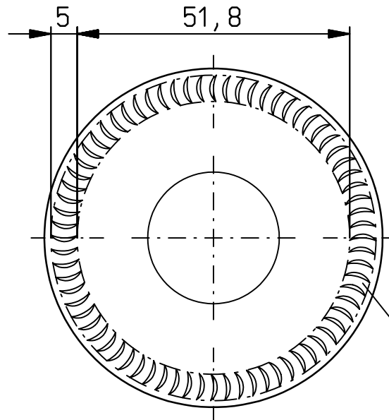
Bodenansicht
