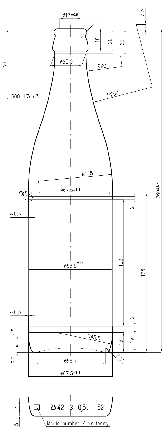
Front view / Widok z przodu
