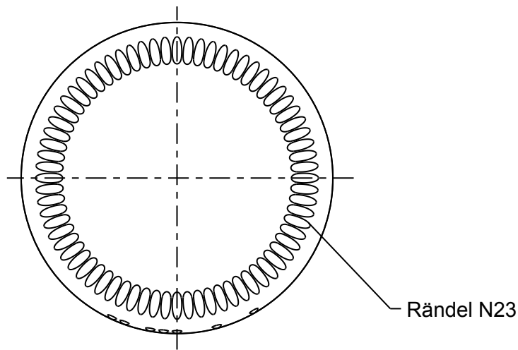
Bodenansicht
